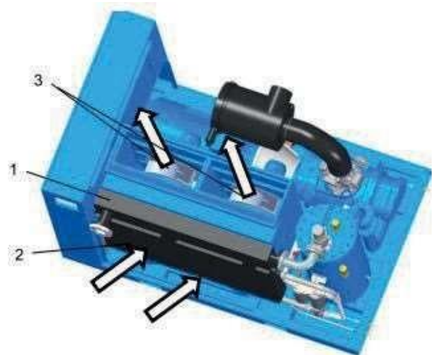
Рис. 15: Вентилятор охлаждения
