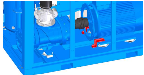
Рис. 29: Транспортный фиксатор
