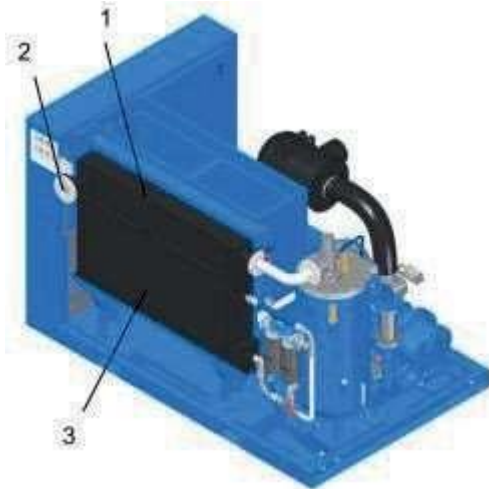
Рис. 12: Охладитель
