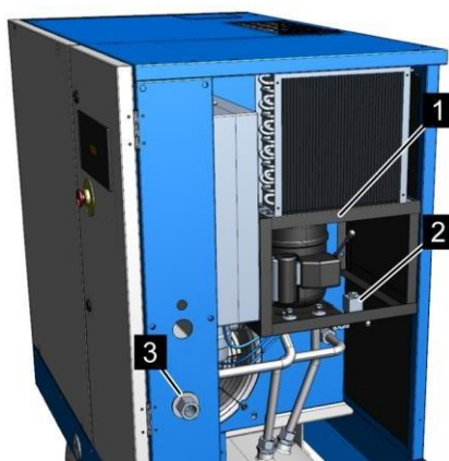
Рис. 23: Рефрижераторный осушитель
