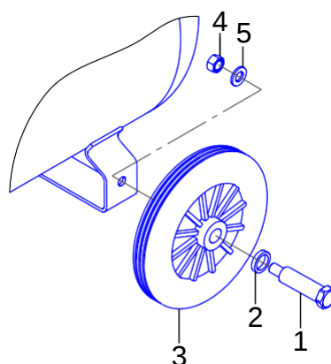
1 - Болт
