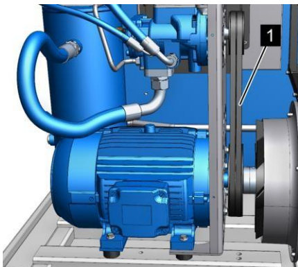
Рис. 15: Приводной агрегат
